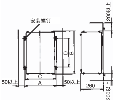
外形图2
