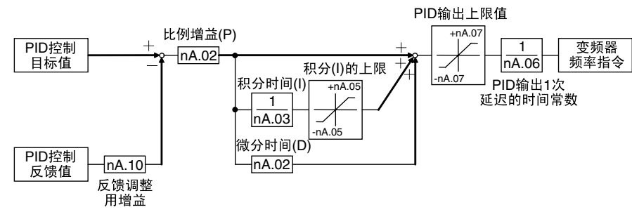
6-4-3 PID 控制模块图
