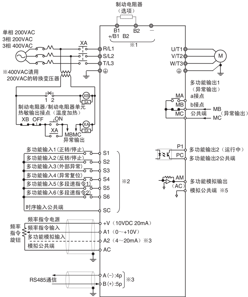
2-2-3 标准配线图
