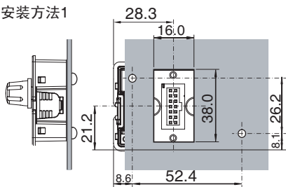
安装方法1
