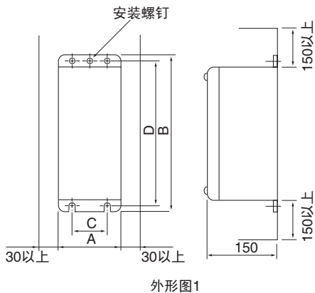
外形图1
